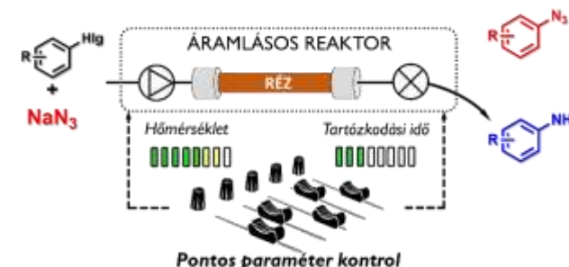
1. ábra: Aril azidok és anilin származékok áramlások szintézise precíz paraméter kontroll által.
