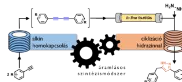
3. ábra: 3,5-diszubsztituált pirazolok szintézise kétlépéses áramlások rendszerben.
