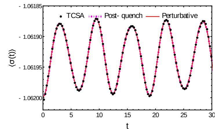
2. ábra: A mágneszettség időfejlődése az Ising térelméletben.
