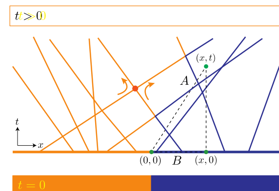
1. ábra: Két rendszer összeillesztése és a szemiklasszikus részecskekép.
