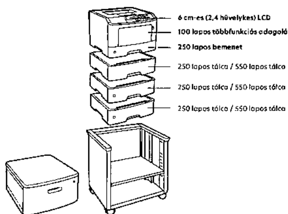
Állítható nyomtatóállvány
